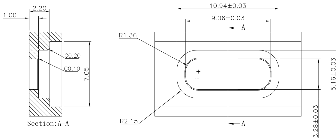
机壳开孔建议尺寸图 \triangle B
